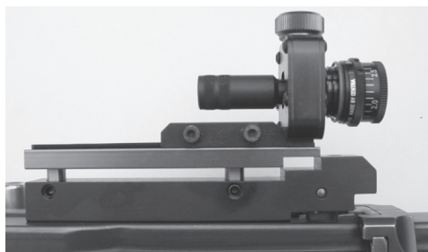
Figure 27: Porte dioptrique pour F ass 57 pour le montage de dioptrique à l'épreuve des vibrations de tir produits divers
